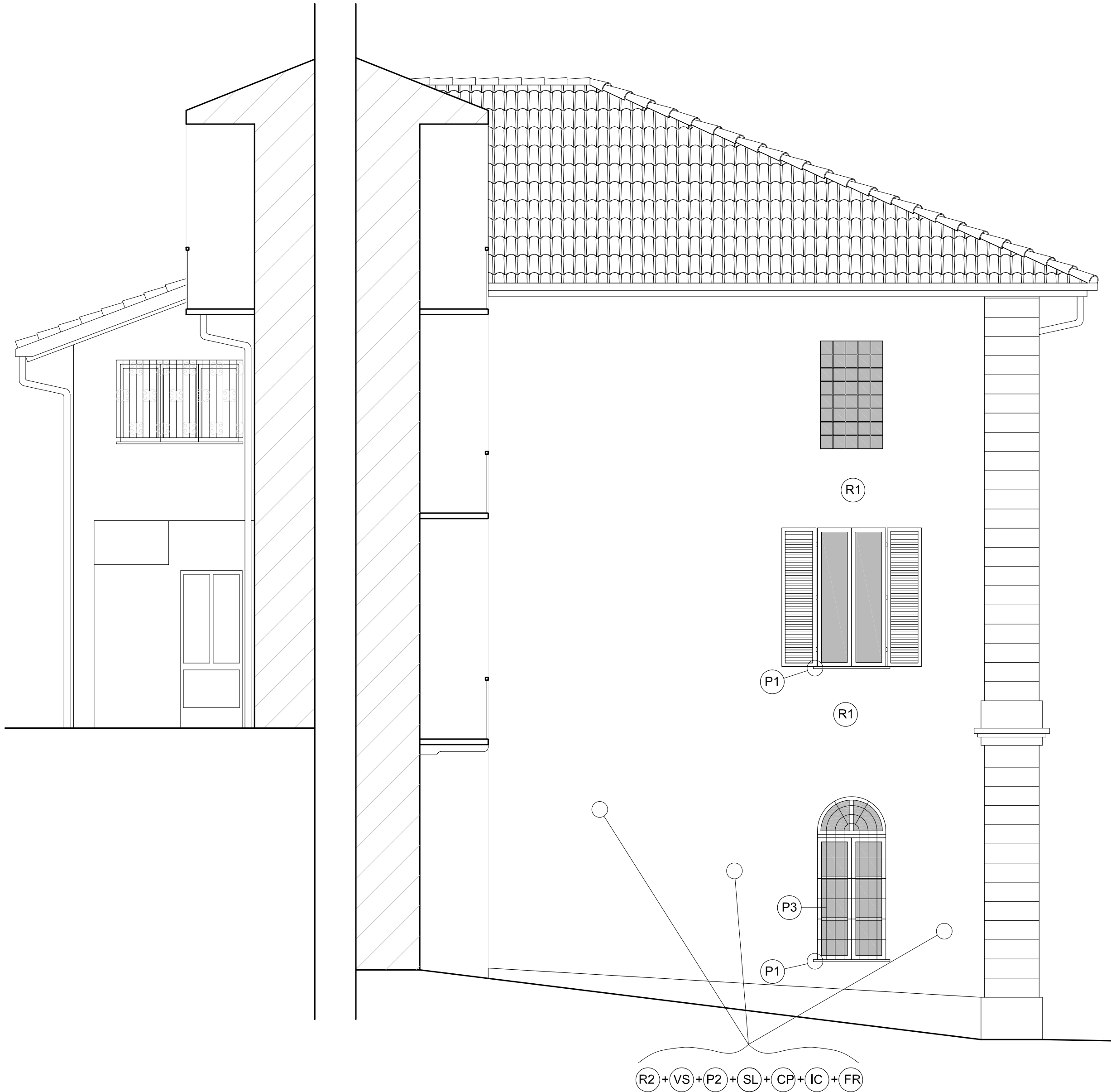
PROSPETTO NORD - OVEST
