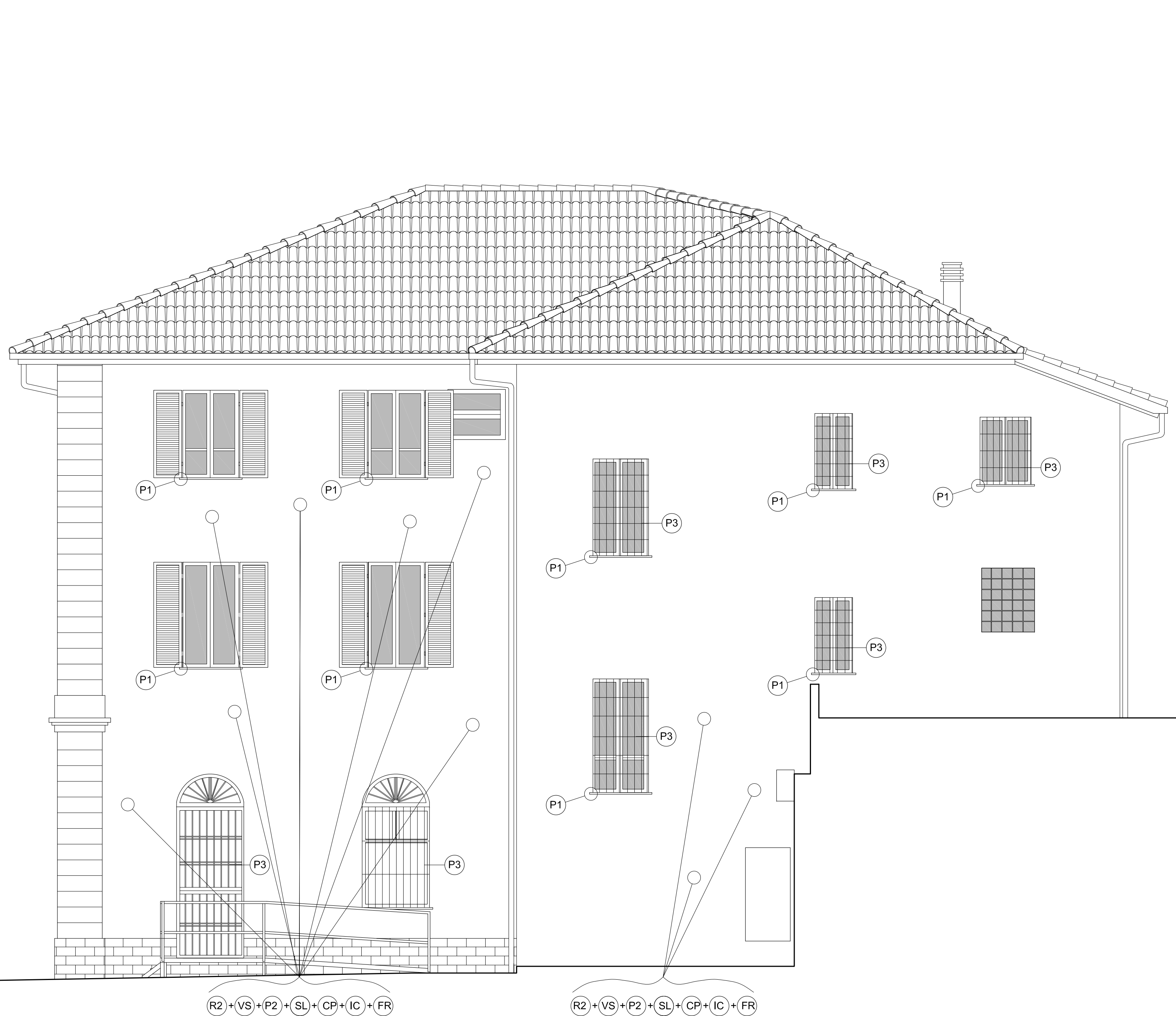
PROSPETTO SUD-EST
