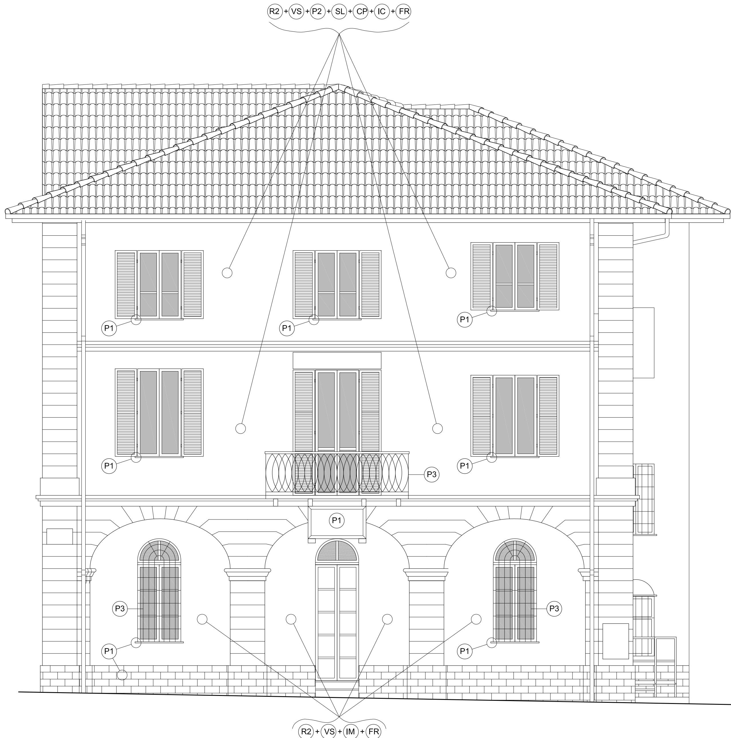
FACCIATA PRINCIPALE - PROSPETTO SUD - OVEST
